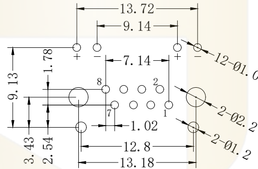
PCB参考图
